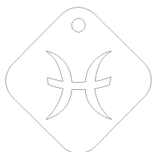
Poisson
