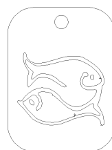
Poisson
